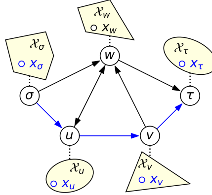
Hình 4.11: Minh họa bài toán SPP in GCS. Mỗi đỉnh i \in \{\sigma, u, v, w, \tau\} trong đồ thị được liên kết với một biến liên tục x_i nằm trong một tập lỗi tương ứng \mathcal{K}_i . Trọng số của mỗi cạnh là một hàm lỗi của các biến liên tục tại hai đỉnh mà cạnh đó kết nối. Trong hình, đường đi màu xanh p = (\sigma, u, v, \tau) thể hiện một nghiệm khả thi của thành phần rời rạc, trong đó tổng chi phí phụ thuộc vào các giá trị tối ưu của x_\sigma, x_u, x_v, x_\tau nhưng độc lập với x_w [16].
